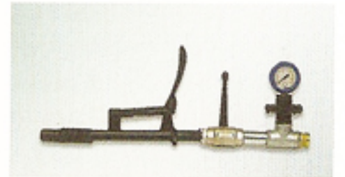
Lança para injeções de cimento com manómetro
